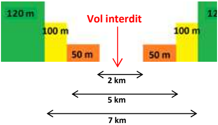
Vue transversale
