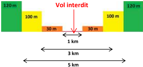
Vue transversale
